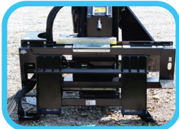
Hydraulic side shift 0" — 26"
